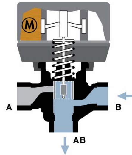
Режим отопления
