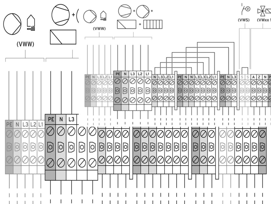
Одноконтурное электропитание
