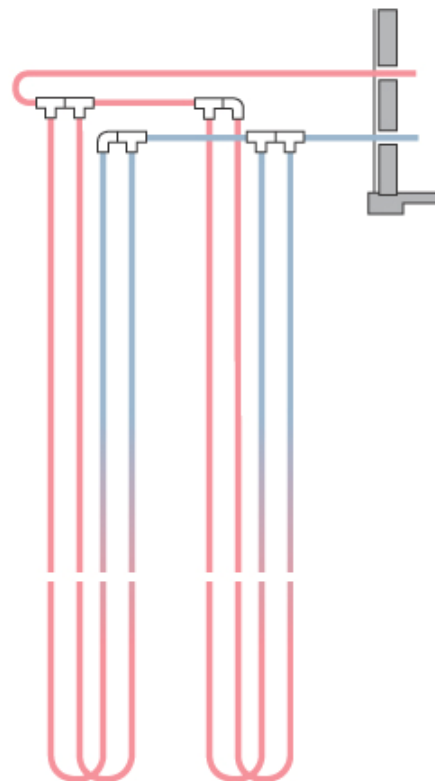
По Тихельманну
