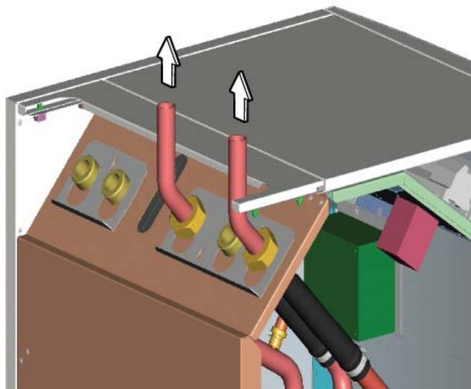
Присоединение вверх
