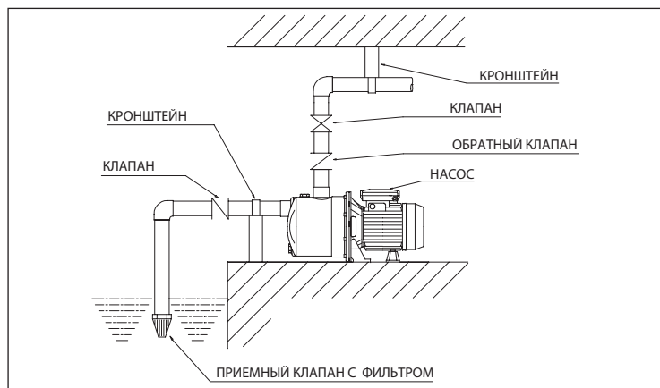
РАЗРЕЗ JEX
