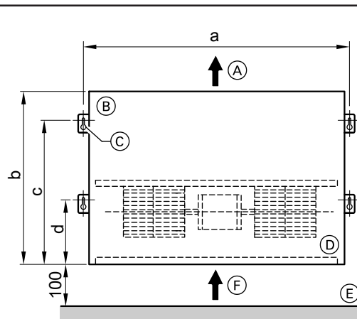
Стеновое крепление (вид спереди)
