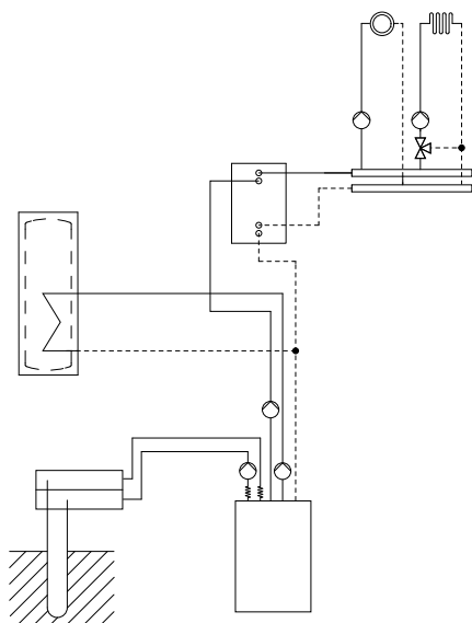
Схема установки 6b: отопительный контур без смесителя A1, отопительный контур со смесителем M2, емкостной водонагреватель, буферная емкость отопительного контура
