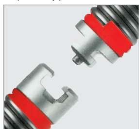
Самоподстраивающееся соединение спирали и муфты
