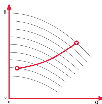
Обеспечение рабочей кривой системы
