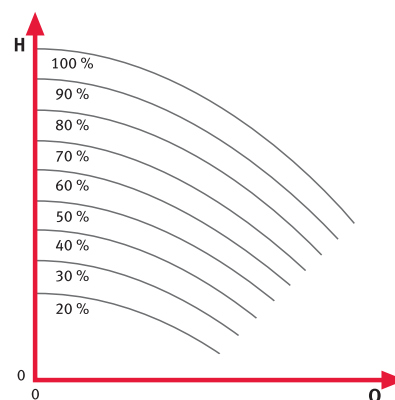
Работа в режиме "исполнительный механизм"
