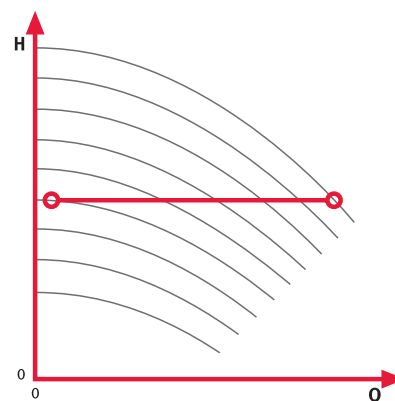
Поддержание постоянного давления
