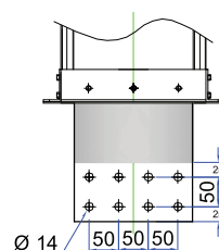
Fig. 4 BUSBAR WIDTH 200 ~ 230mm
