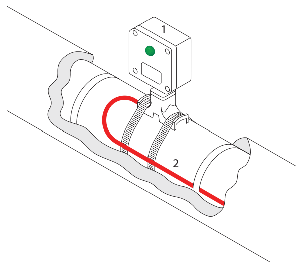
1 – соединительная коробка РТВ 401-ИС 2 – нагревательная секция (лента)
