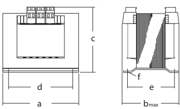
Maßbild Dimensions Габаритный чертёж
