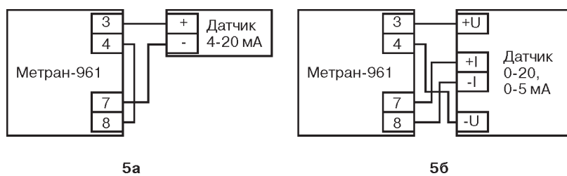
Рис.5. Подключение датчиков по 2-х-проводной (5а) и 4-х-проводной (5б) схемам.
