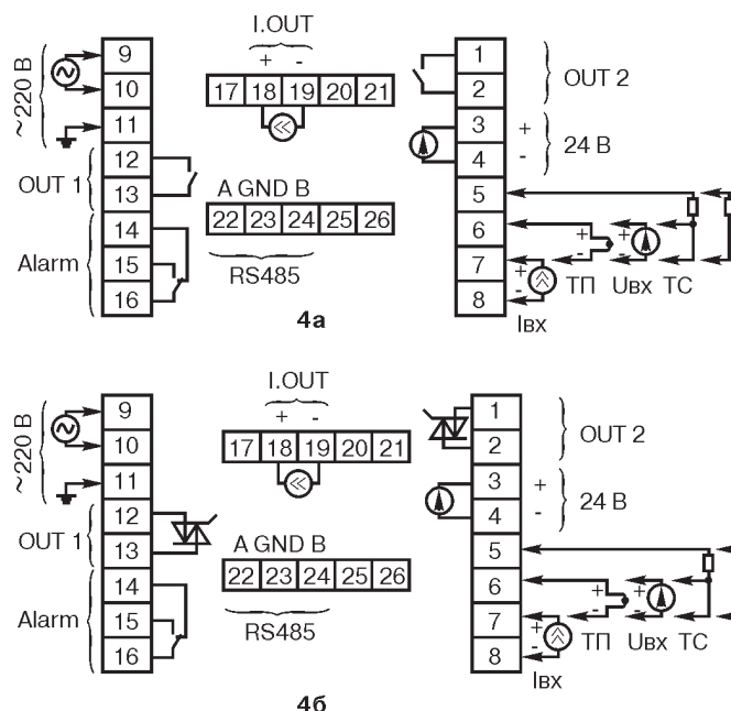
Рис.4. Расположение и назначение клемм прибора.
