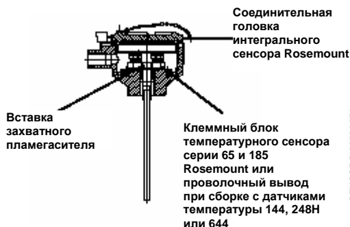
РИСУНОК 4. Конфигурация взрывозащиты ATEX/CENELEC
