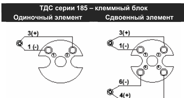
РИСУНОК 3. Конфигурация соединения проводов ТДС серии 185
