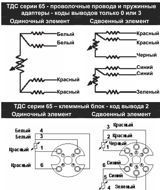
РИСУНОК 2. Конфигурация соединения проводов ТДС серии 65
