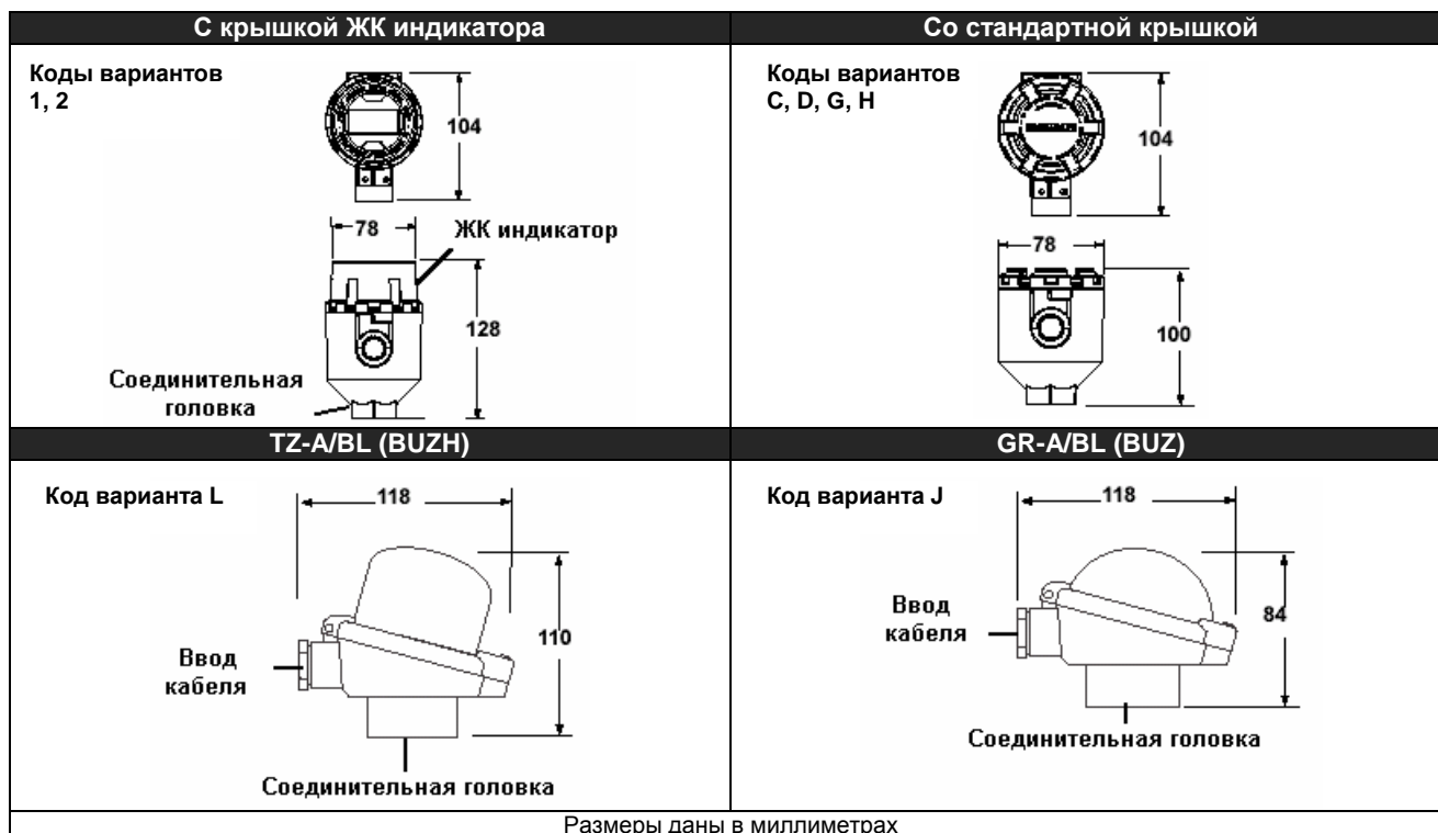
РИСУНОК 5. Габаритный чертёж соединительной головки
