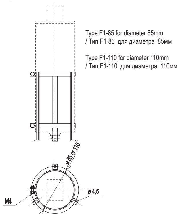
Clamp type F... / Держатель типа F...
