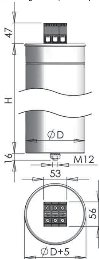
Drawing No./Габаритный чертёж 3b
