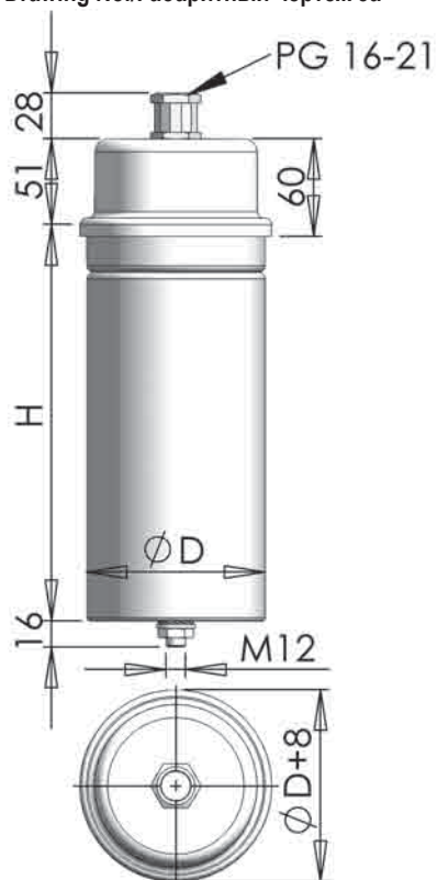
Drawing No./Габаритный чертёж 3a
