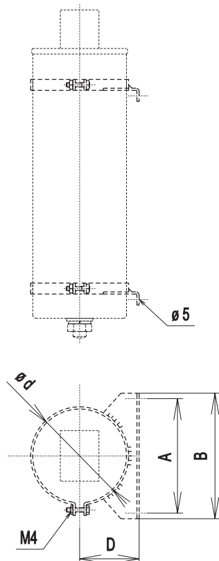
Clamp type A... / Держатель типа А...
