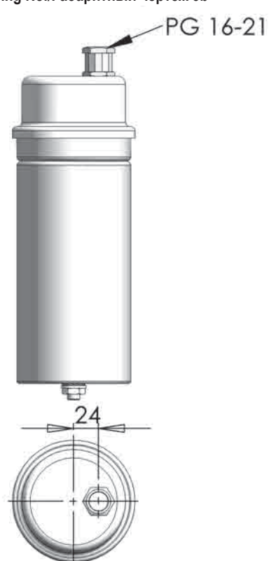
Drawing No./Габаритный чертёж 3b
